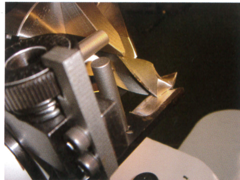
▲ Drill Positioning Device ドリル位置取り装置
