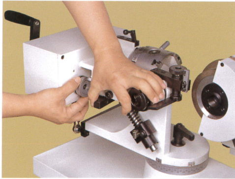
▲ Cam Device カム取り替え
